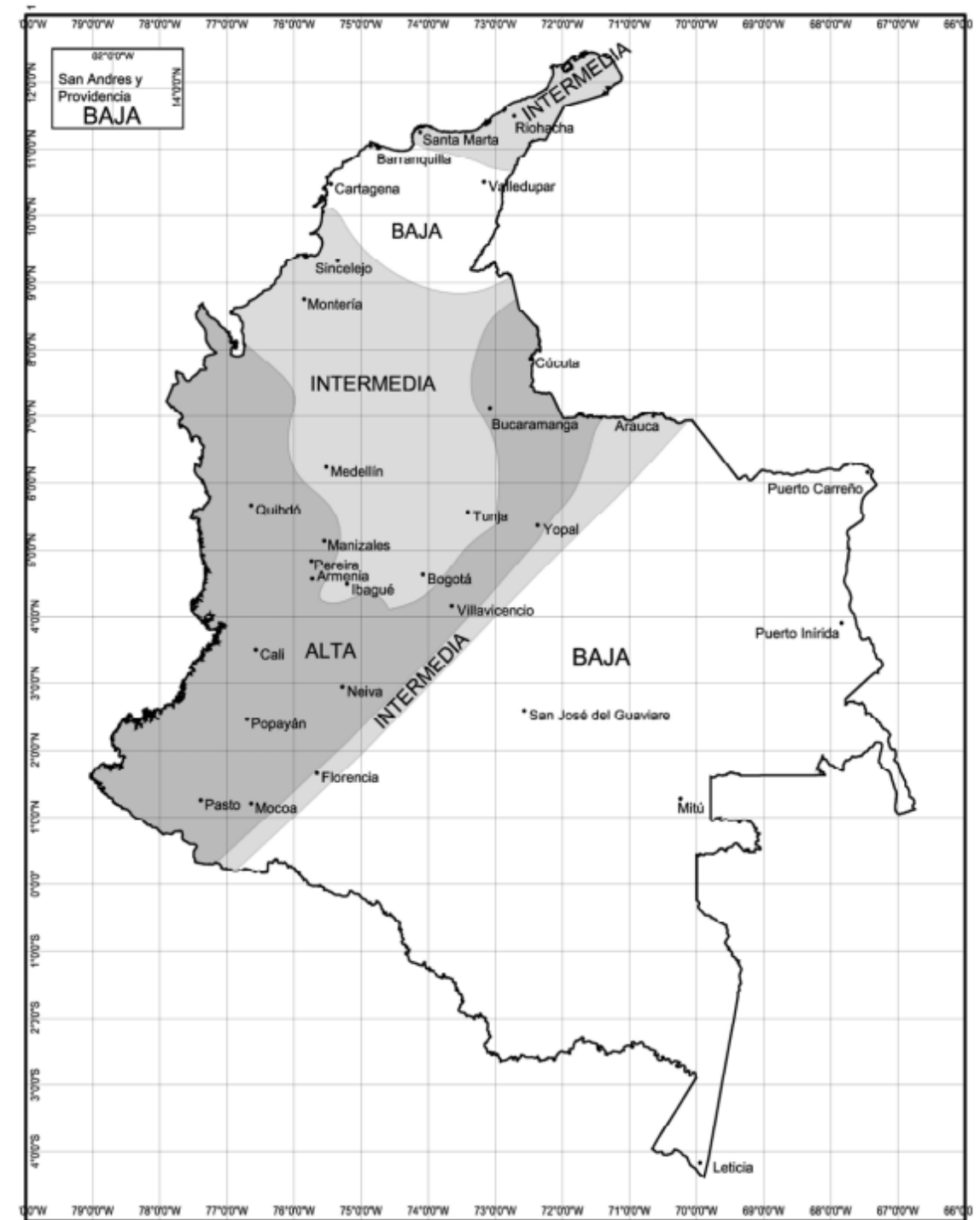
Figura 3. Zonas de Amenaza Sísmica en Colombia.
